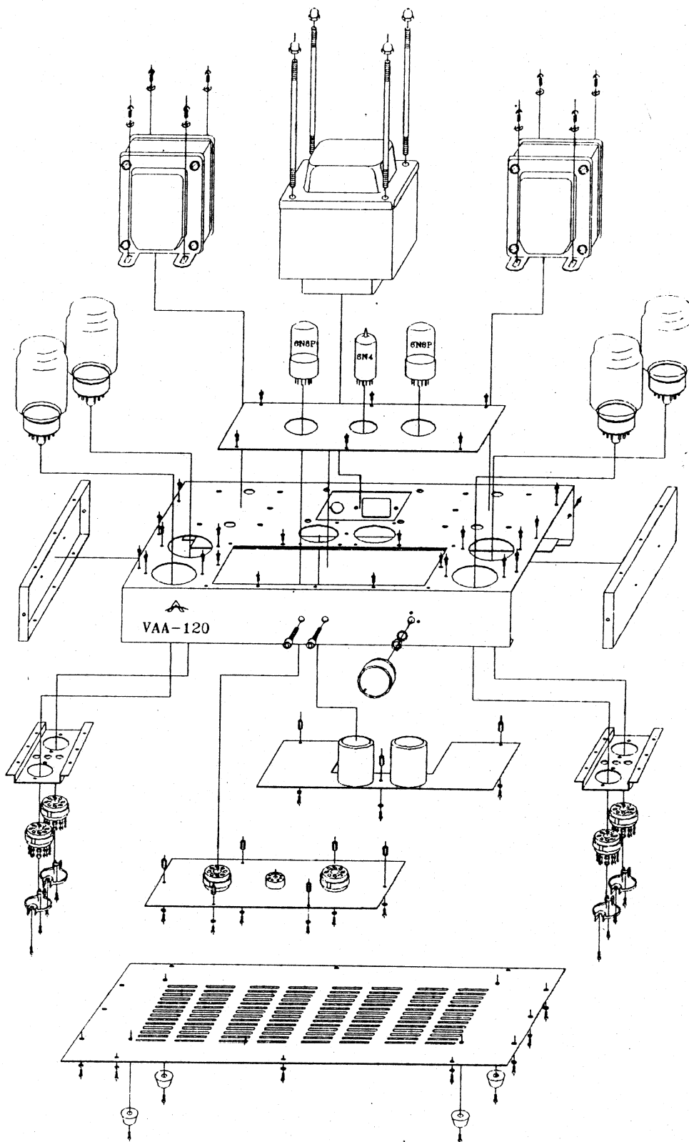
VAA-120結構裝配總圖
